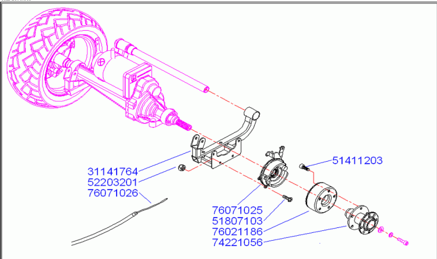
名稱：手煞車組合 圖號：S800M302 核准 版次：0 日期2009/04/15
